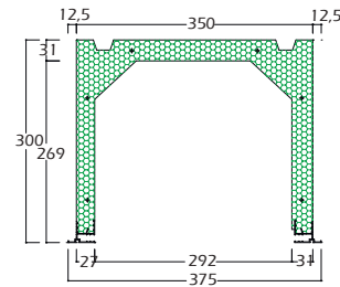
Cassonetto EUR 35
