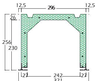
Cassonetto EUR 30/25
