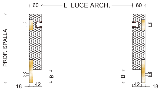
Senza Rivestimento
