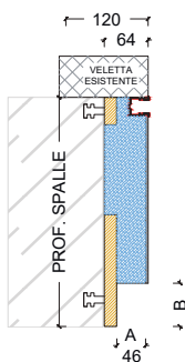
Per Ristrutturazione
