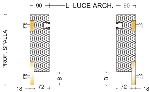
Senza Rivestimento
