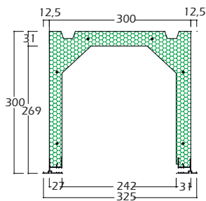
Cassonetto EUR 30
