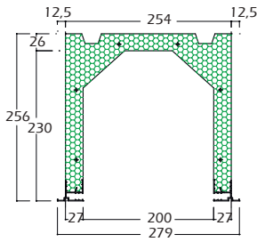
Cassonetto EUR 25
