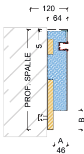
Installazione Standard
