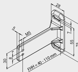
Squadretta per guide in ghisa cod. tipo 2
