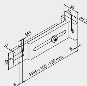
Squadretta per guide tipo 4
