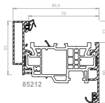
Profilo anta finestra complanare
