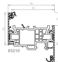
Profilo anta finestra a gradino
