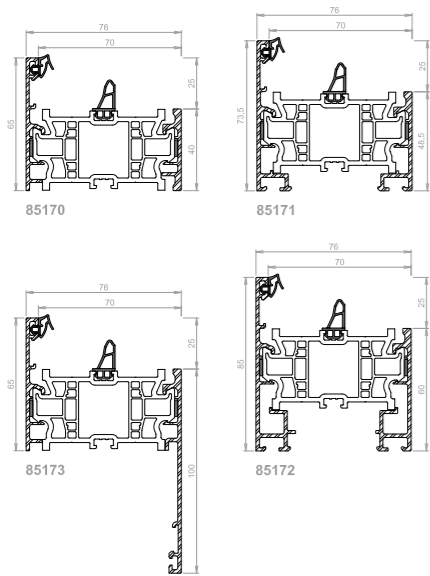
Telai per sistema a 3 guarnizioni
