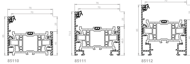
Telai per sistema a 2 guarnizioni
